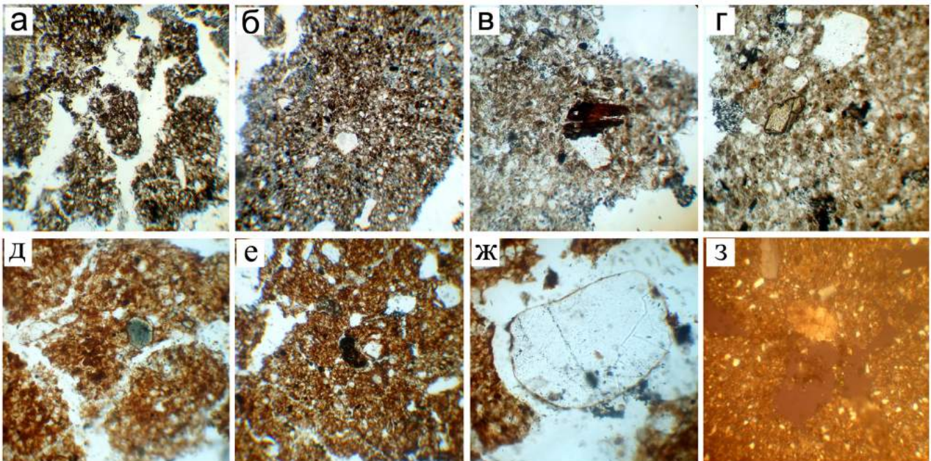
Рисунок 3. Мікроморфологічні особливості гумусових горизонтів (Н і Нк): а) темно-сіра пилювато-плазмова елементарна мікробудова Н горизонту (орного шару) з гумусово-глинистою плазмою, мікроагрегатами високого порядку (до IV), розвинутою системою між- і внутрішньоагрегатних звивистих пор /зб. 70, нік. II/; б) добра гумусованість маси Н горизонту, пилювато-плазмова мікробудова /зб. 140, нік. II/; в) напіврозкладені рештки рослини в Н горизонті /зб. 140, нік. II/; г) первинні мінерали у складі мінерального скелету Н горизонту представлені, крім пилюватих зерен кварцу, польовими шпатами, слюдою та іншими мінералами /зб. 140, нік. II/; д) складні мікроагрегати розділені неправильними каналоподібними порами в Нк горизонті, зерно рогової обманки /зб. 70, нік. II/; е) мікробудова Нк горизонту з сірувато-темно-бурою гумусово-карбонатно-глинистою плазмою, пори неправильної форми, округлі, овальні /зб. 70, нік. II/; ж) піщане зерно кварцу в Нк горизонті /зб. 140, нік. II/; з) пилювато-плазмова елементарна мікробудова Нк горизонту, просочення маси мікрокристалічним кальцитом /зб. 70, нік. +/
