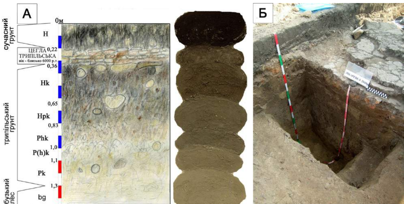
Рисунок 2. Польова зарисовка відкладів шурфа № 1 на пам'ятці Лікарів з розчленуванням на генетичні горизонти та примазками натурального матеріалу (А), фото шурфа (Б)
